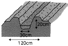
図2 植え付け
